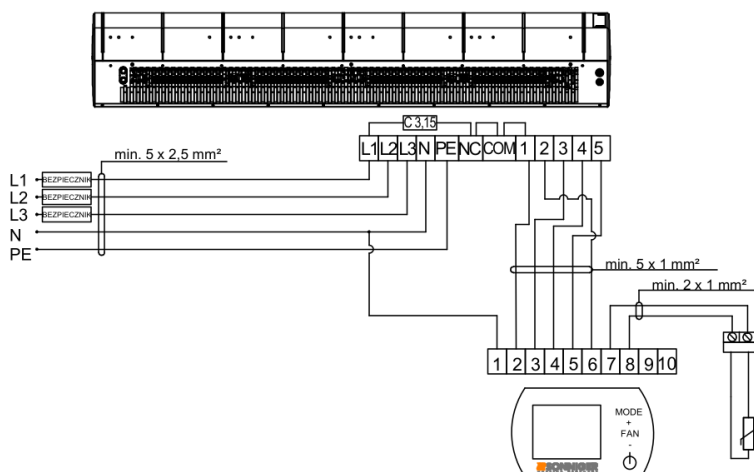
Схема подключения двух завес GUARD 100-150-200E к панели управления INTELLIGENT
